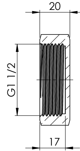
SCHNITT A-A
